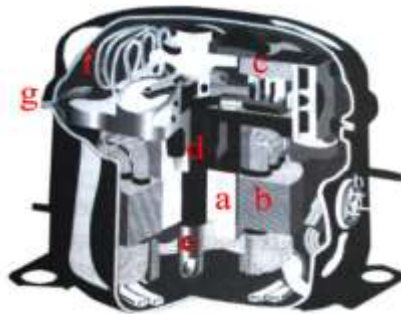
Gambar Kompresor Jenis Hermetik
