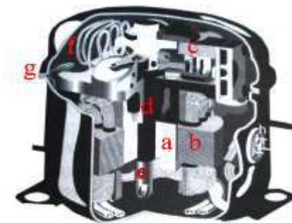
Gambar Kompresor Jenis Hermetik
