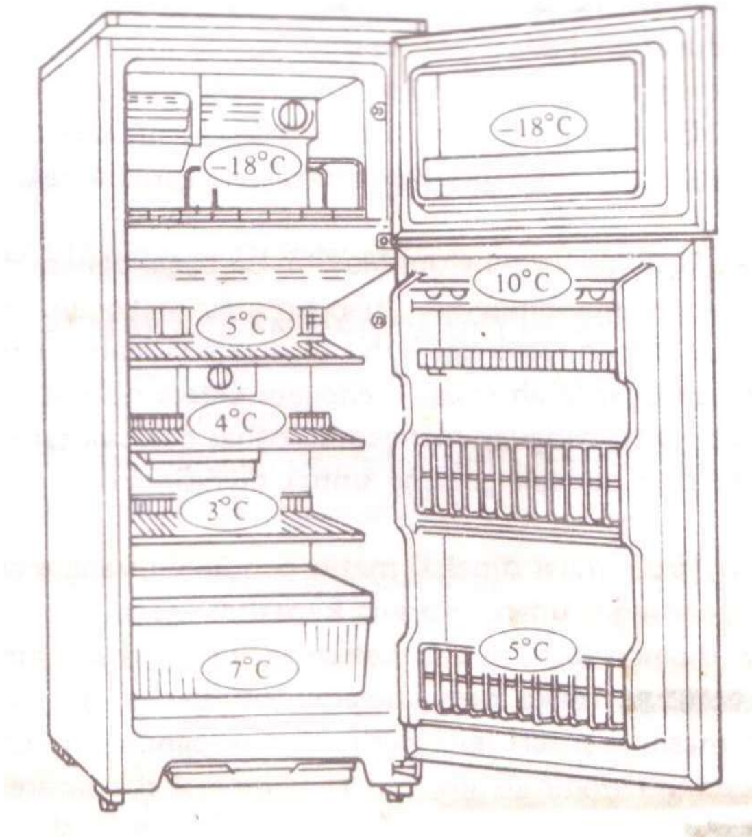
Gambar. Distribusi Temperatur di Dalam Kompartmen Kulkas
