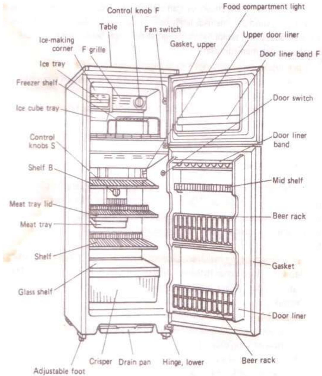
Gambar. General Bagian Dalam Kulkas
